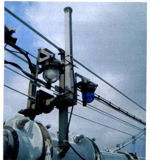
Станция спутникового мониторинга висячего моста Tsing Ma в Китае
